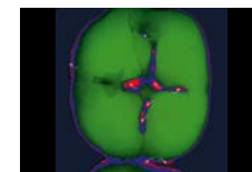
Funkce Proof
